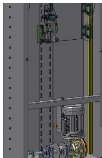
B) SMAROWANIE PROWADNIC KOLUMNY
